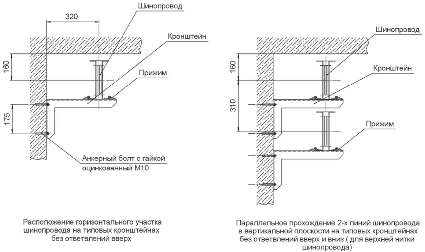
Рисунок 8 - Горизонтальное расположение однопакетных шинопроводов на типовых кронштейнах
