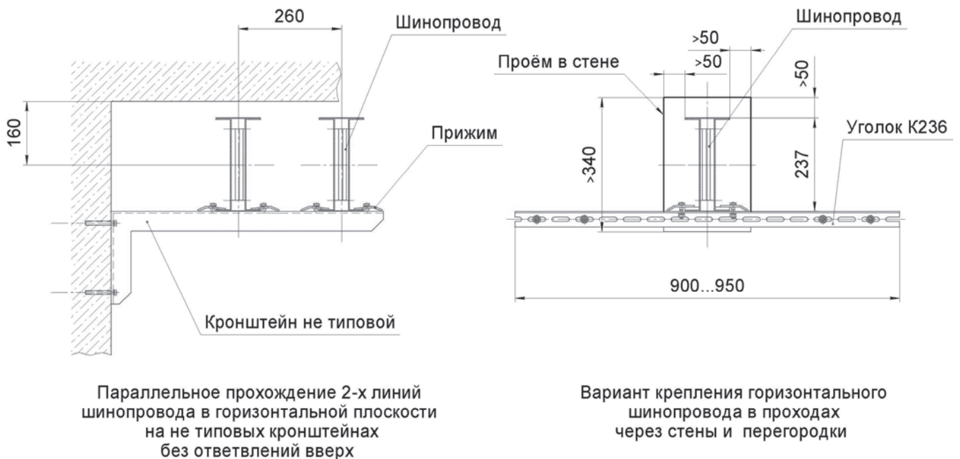
Рисунок 9 - Горизонтальное расположение однопакетных шинопроводов на не типовых кронштейнах, проход через стену
