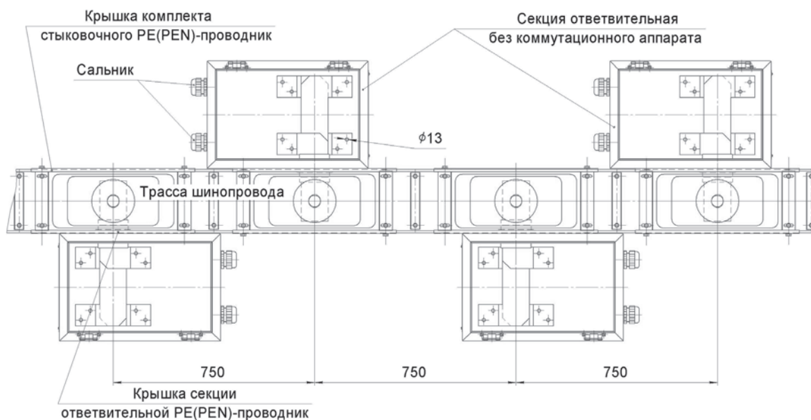
Рисунок 2 - Пример установки коробок ответвительных
