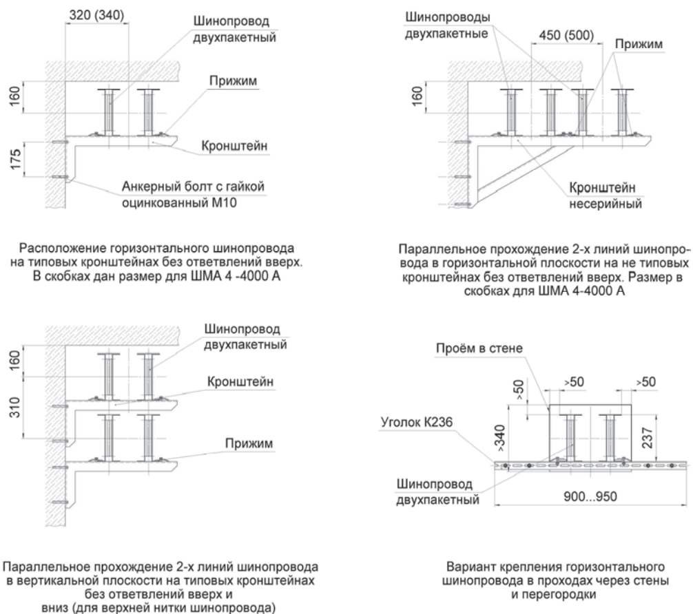
Рисунок 11 - Горизонтальное расположение двухпакетных шинопроводов на типовых и не типовых кронштейнах, проход через стену
